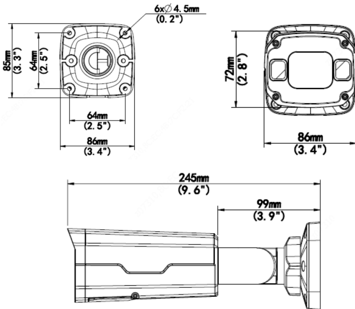
XLGUP06-C Montage sur Poteau
